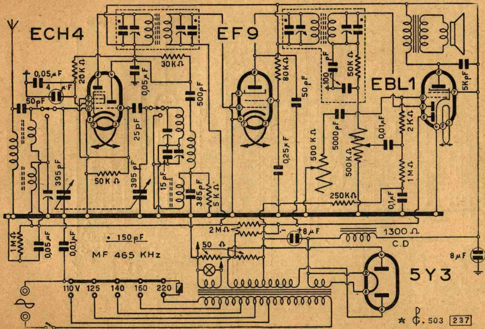
Lo schema elettrico del mod. Sicilia
